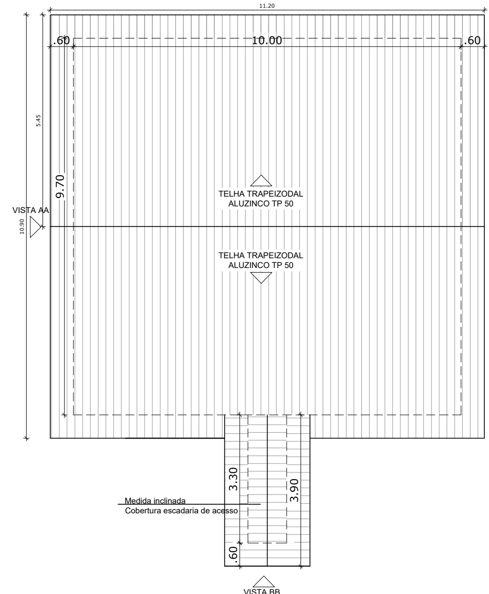
PLANTA DE COBERTURA Esc.:1/100
